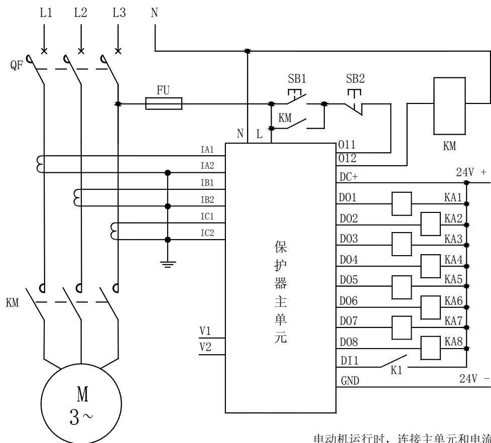
AMDG-X/F5□1 系列电动机保护器 DO 连接继电器电气原理图
