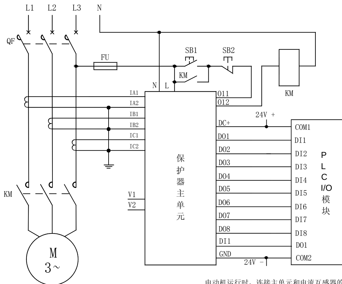
AMDG-X/F5□1 系列电动机保护器 D0 连接 PLC 电气原理图
