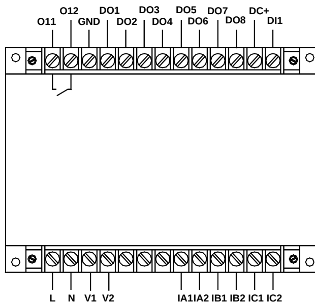
AMDG-X/F5□1 系列保护器主单元端子图
