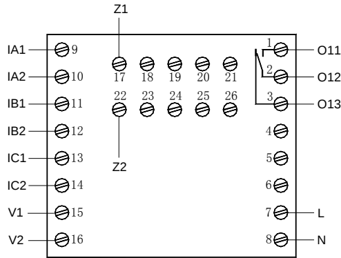
AMDP-□/D011 系列保护器主单元端子图
