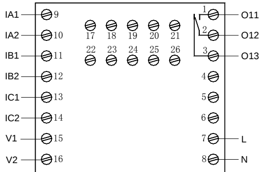
AMDP-□/D001 系列保护器主单元端子图
