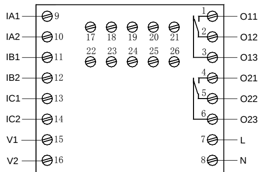
AMDP-□/D002 系列保护器主单元端子图
