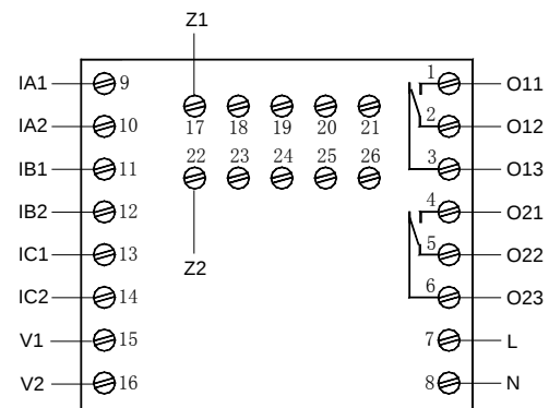
AMDP-□/D012 系列保护器主单元端子图
