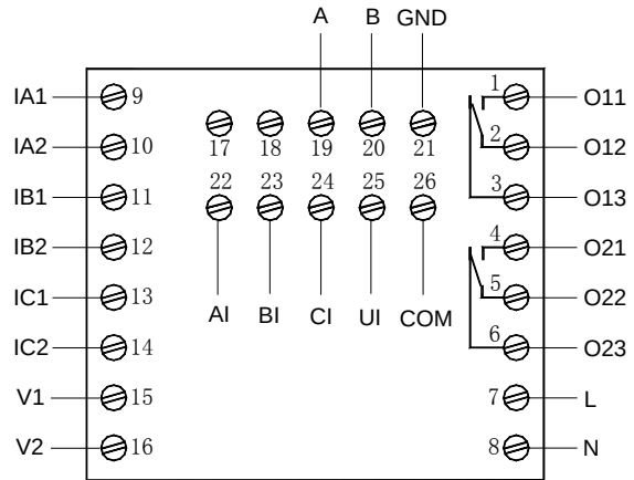
AMDP-□/D4□2 系列保护器主单元端子图
