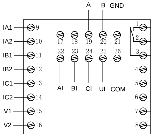
AMDP-□/D4□1 系列保护器主单元端子图
