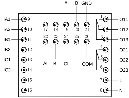
AMDP-X/E402 系列保护器主单元端子图
