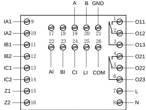
AMDP-X/E412 系列保护器主单元端子图
