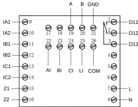
AMDP-X/E411 系列保护器主单元端子图
