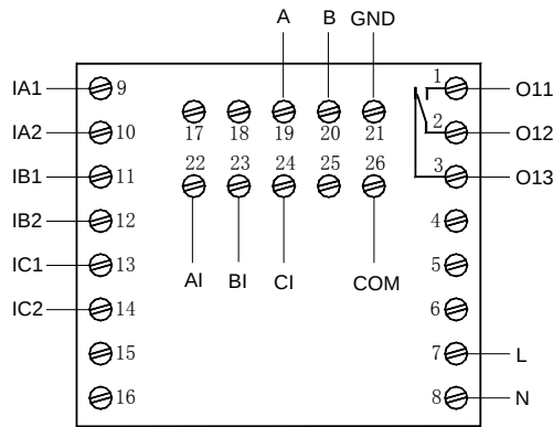
AMDP-X/E401 系列保护器主单元端子图
