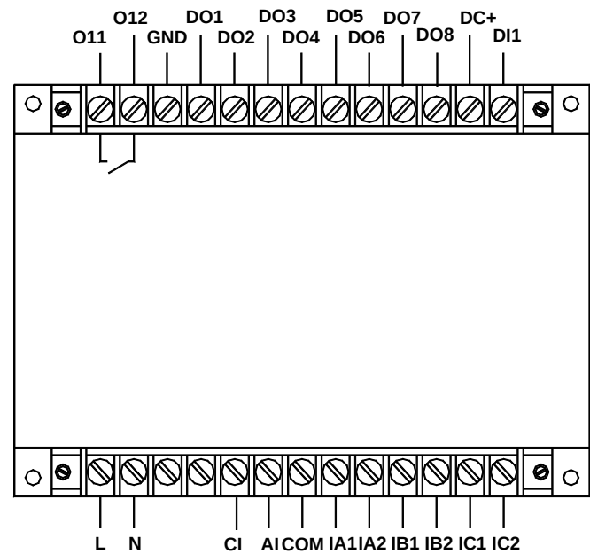
AMDG-□/701 系列保护器主单元接线端子图
