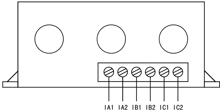
AMDG-□/701 系列保护器电流检测单元接线端子图
