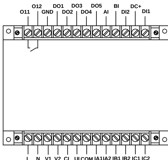
AMDG-X/F841 系列保护器主单元接线端子图
