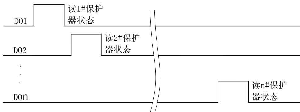
PLC 读取多台 AMDG-X/F841 系列电动机保护器时序图
