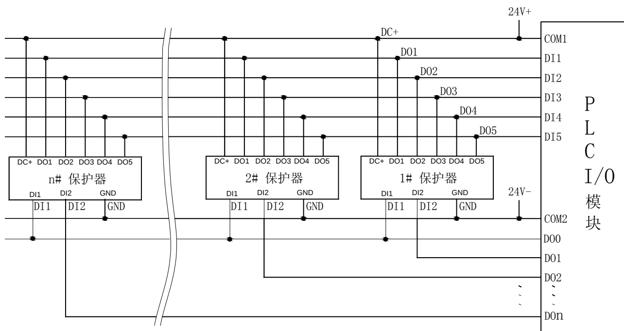
PLC 读取多台 AMDG-X/F841 系列电动机保护器电气原理图
