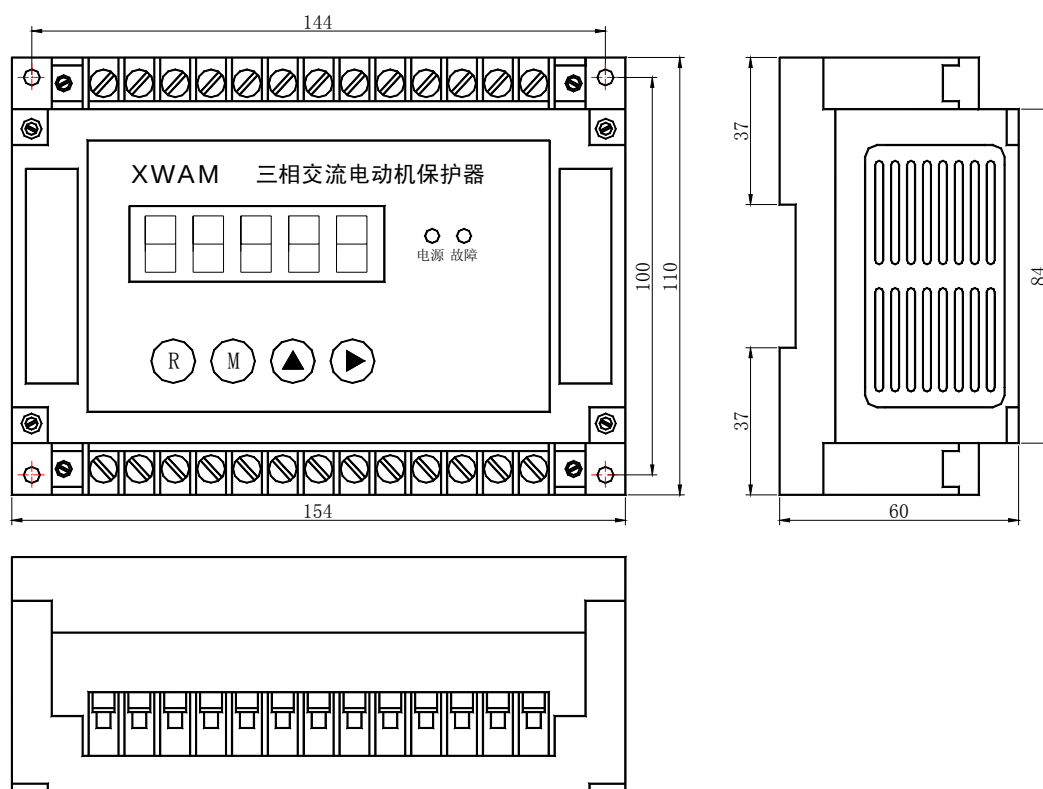
AMDG-X/F841 系列电动机保护器主单元外形及安装孔尺寸
